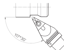
MCD' HSK-A63 F.77 SVVBN 140.16
