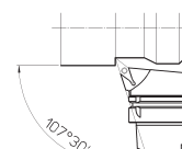
MCD' HSK-A63 F.26 SVHBR/L 065.16
