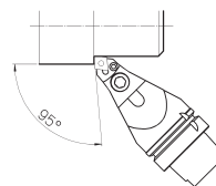
MCD' HSK-A63 F.77 PCMNN 130.12
