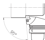
MCD' HSK-A63 F.26 PCLNR/L 065.12
