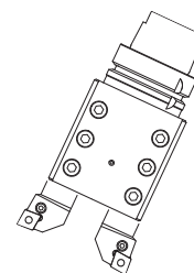
MCD' HSK-A63 TU 25.02
