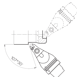
MCD' HSK-A63 F.77 PDNNN 140.15
